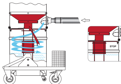
Opcjonalny pływak do systemu zbierania cieczy
